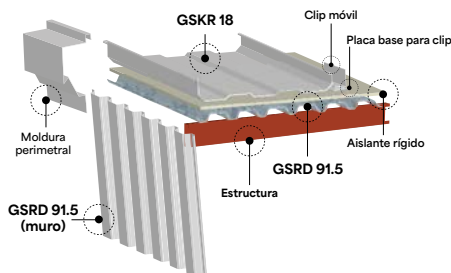
Cubierta compuesta GSRD 91.5 y GSKR 18
