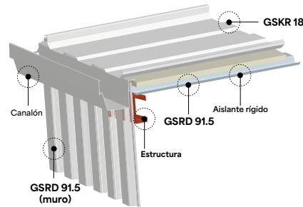
Solución en zona de canalón
