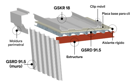
Cubierta compuesta GSRD 91.5 y GSKR 18 Muro GSRD 91.5
